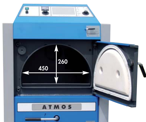
Velikost příkladací komory
